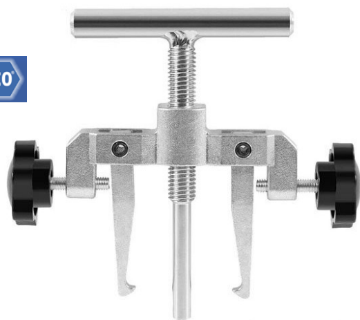
24.0195007004 Estrattore (Tool) 40 - 65 mm 24.0195007020 Estrattore (Tool) 65 - 118 mm
